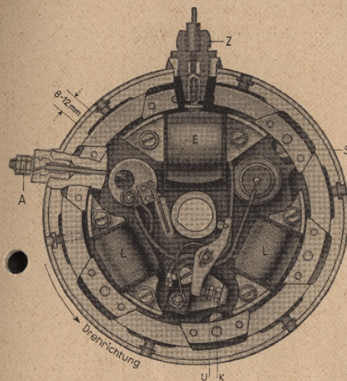
E: Zündspule L: Lichtspule S: Stellschrauben f. d. Grundplatte A: Anschluß für Lichtkabel Z: Anschluß f. Zündkabel U: Unterbrecher K: Feststellmutter
