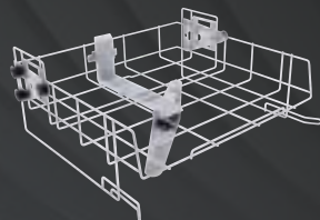
Höhenverstellbarer Oberkorb mit eingebautem Spülarm (A 102)
